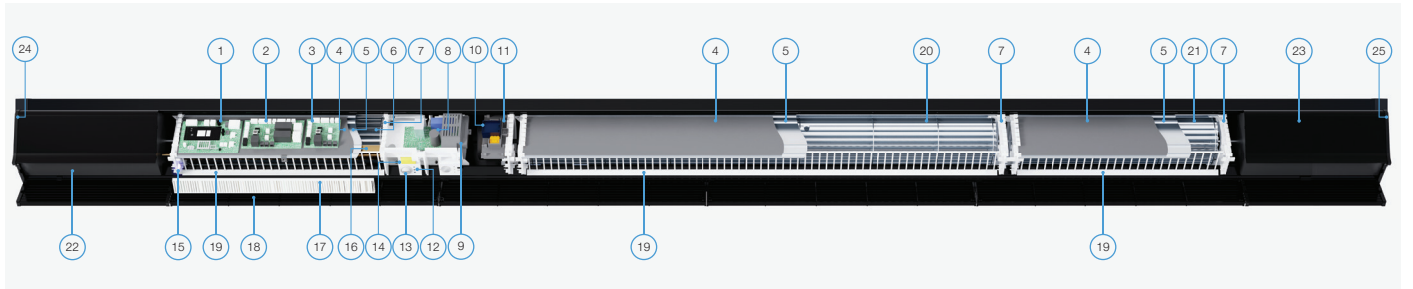
Şek. 3-3-2 Core 2 Pure Serisi Cihaz Modülleri / Ön Kısım
