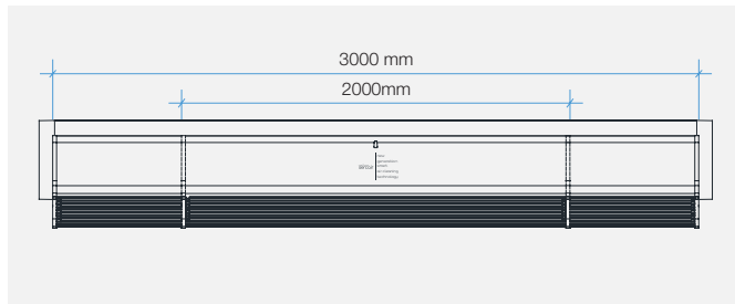
Şek. 3-3-1-1 Cihaz Teknik Detay
