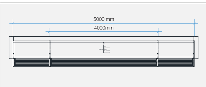
Şek. 3-5-1-1 Cihaz Teknik Detay
