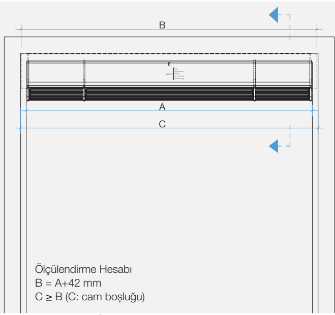
Şek. 3-6-1 Sercair Core Pure Serisi Ölçülendirme Detayları
