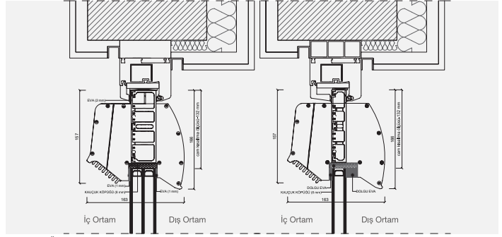
Şek. 3-6-2 Üçlü Cam Kesiti
