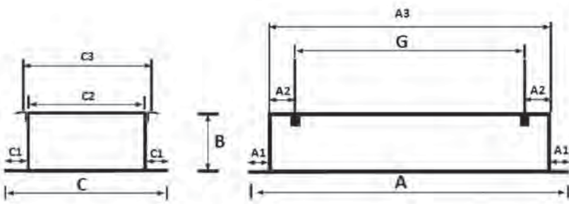
ANKASTRE TİCARİ TİP SU VE BUHAR SERPANTİNLİ HAVA PERDELERİ EBAT VE AĞIRLIK TABLOSU
