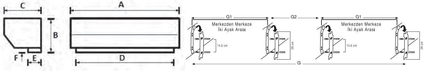
ENDÜSTRİYEL TİP ISITICISIZ HAVA PERDELERİ EBAT VE AĞIRLIK TABLOSU
