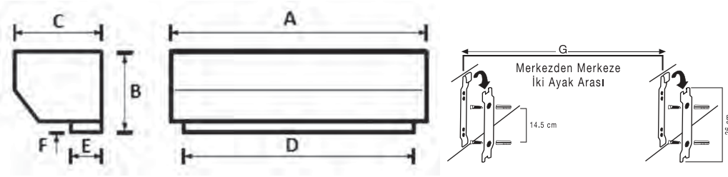
GENEL TİP S SERİSİ ELEKTRİKLİ ISITICILI HAVA PERDELERİ EBAT VE AĞIRLIK TABLOSU
