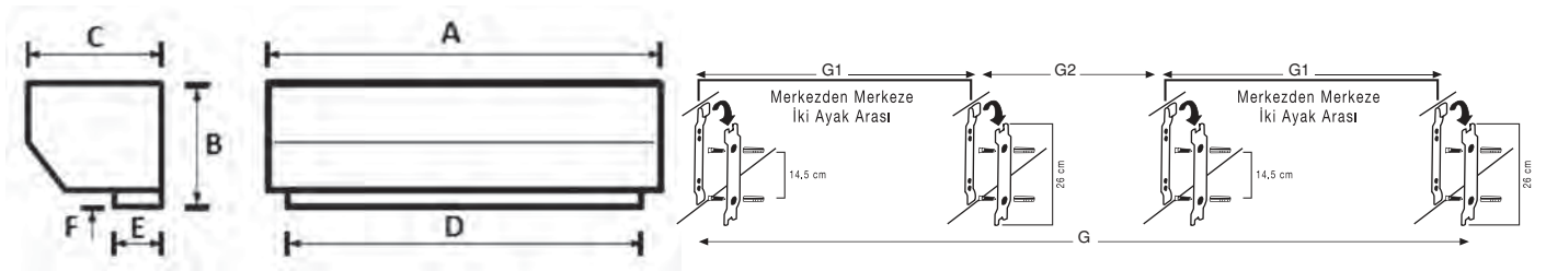
ENDÜSTRİYEL TİP ELEKTRİKLİ ISITICILI HAVA PERDELERİ EBAT VE AĞIRLIK TABLOSU
