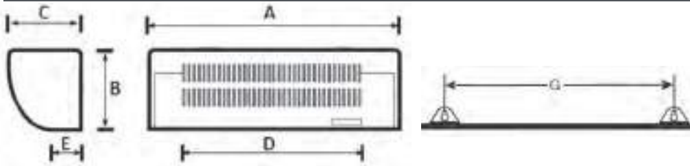
GENEL TİP INOX SERİSİ ISITICISIZ HAVA PERDELERİ EBAT VE AĞIRLIK TABLOSU
