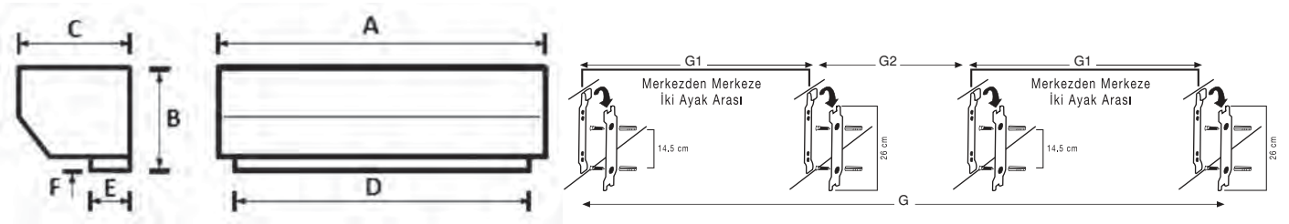
GENEL TİP ELEKTRİKLİ ISITICILI HAVA PERDELERİ EBAT VE AĞIRLIK TABLOSU
