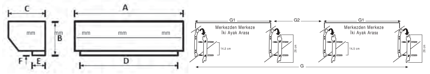
ENDÜSTRİYEL TİP SU VE BUHAR SERPANTİNLİ HAVA PERDELERİ EBAT VE AĞIRLIK TABLOSU
