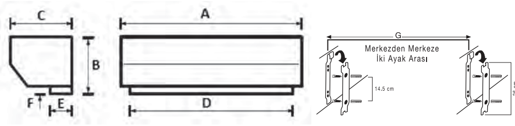
GENEL TİP INOX SERİ ELEKTRİKLİ ISITICILI HAVA PERDELERİ EBAT VE AĞIRLIK TABLOSU
