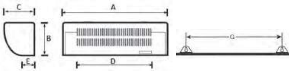
INTELLECT TİP ELEKTRİKLİ ISITICILI HAVA PERDELERİ EBAT VE AĞIRLIK TABLOSU
