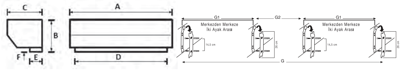
TİCARİ TİP ELEKTRİKLİ ISITICILI HAVA PERDELERİ EBAT VE AĞIRLIK TABLOSU
