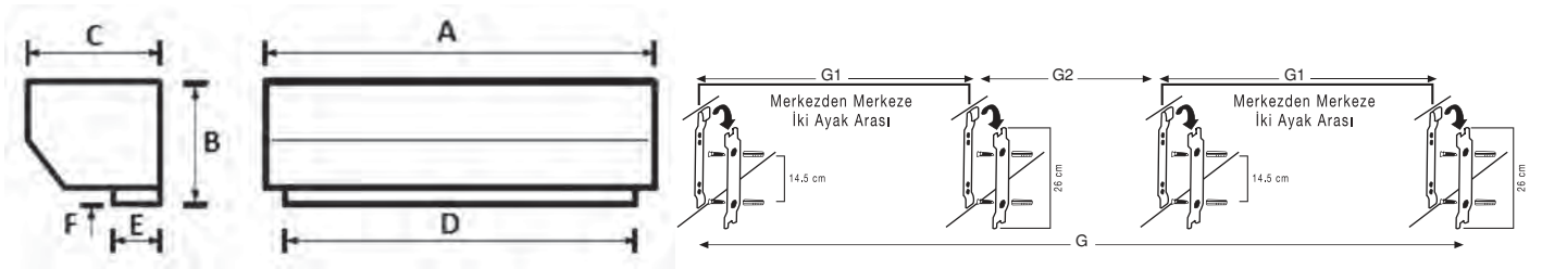
TİCARİ TİP SU VE BUHAR SERPANTİNLİ HAVA PERDELERİ EBAT VE AĞIRLIK TABLOSU
